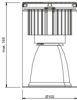
Skizze für 2x25°. Die Höhe ist abhängig vom Reflektor! Sketch for 2x25°. The height depends on the reflector!
